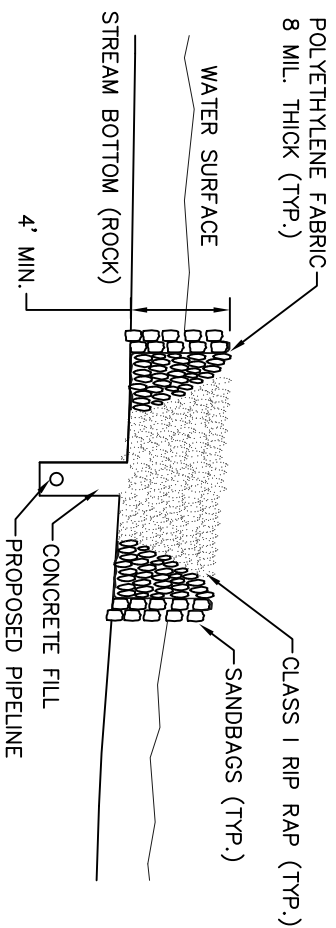
SECTION A-A
